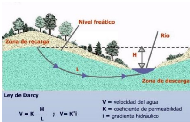
Figura 20. Ley de Darcy
