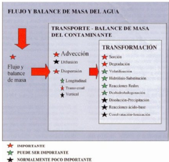
Figura 23. Procesos hidro-Geológicos, que afectan a las aguas subterráneas.
