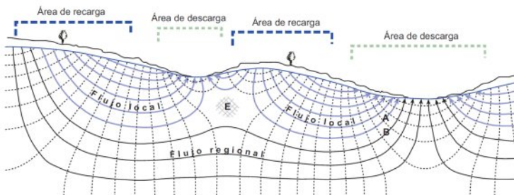
Figura 21. Redes de flujo de agua subterránea
